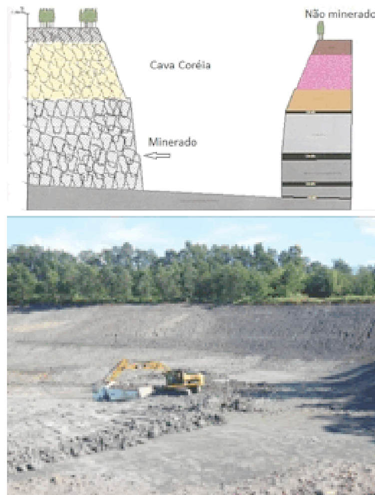
Figura 3a e b.- Perfil das camadas mineradas e não mineradas e deposição planejada de estéreis no “bota-fora”.
