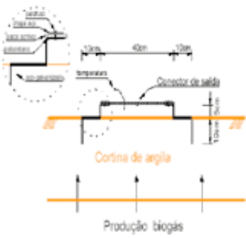
Figura 7a e b – Perfil da placa de fluxo e vedação no contato placa-tampa para medição
