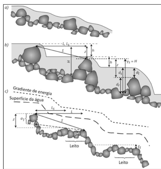
Figura 3 – Unidades geomorfológicas de pequena escala e materiais de leito: (a) canais rápidos; (b) step-pools; e (c) step-pools com interação do leito (Modificado de Church e Zimmermann, 2007).
