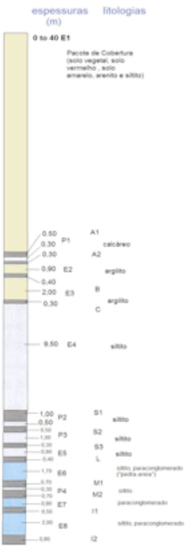
Figura 2 - Perfil estratigráfico mostrando as camadas de carvão
