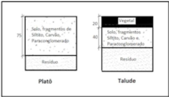
Figura 4a e b - Perfil da camada de cobertura e pedregulhos encontrados no local
