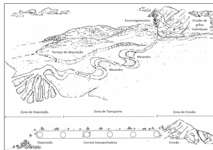
Figura 2 – Produção de sedimentos em rios (Modificado de Kondolf, 1994)
