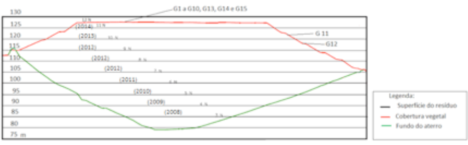
Figura 6 – Perfil das camadas de resíduos e localização dos pontos de medição
